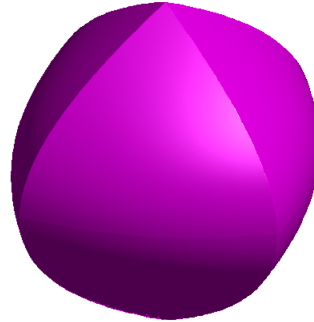
(d) \ell_1/\ell_2 -norm ball: \Omega(\mathbf{w}) = \|\mathbf{w}\|_2 + |\mathbf{w}_1| + |\mathbf{w}_2| .
