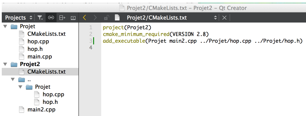
FIGURE 6.2 – Même source dans deux projets : hop.cpp et hop.h sont partagés par les deux projets, même s'ils se trouvent dans le dossier Projet
