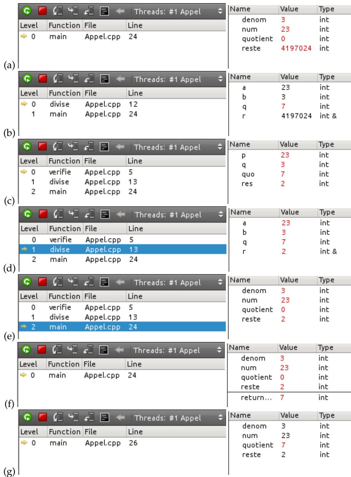
FIGURE 7.1 – Appels de fonctions
