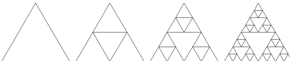
FIGURE A.7 – Construction du triangle de Sierpinski.
